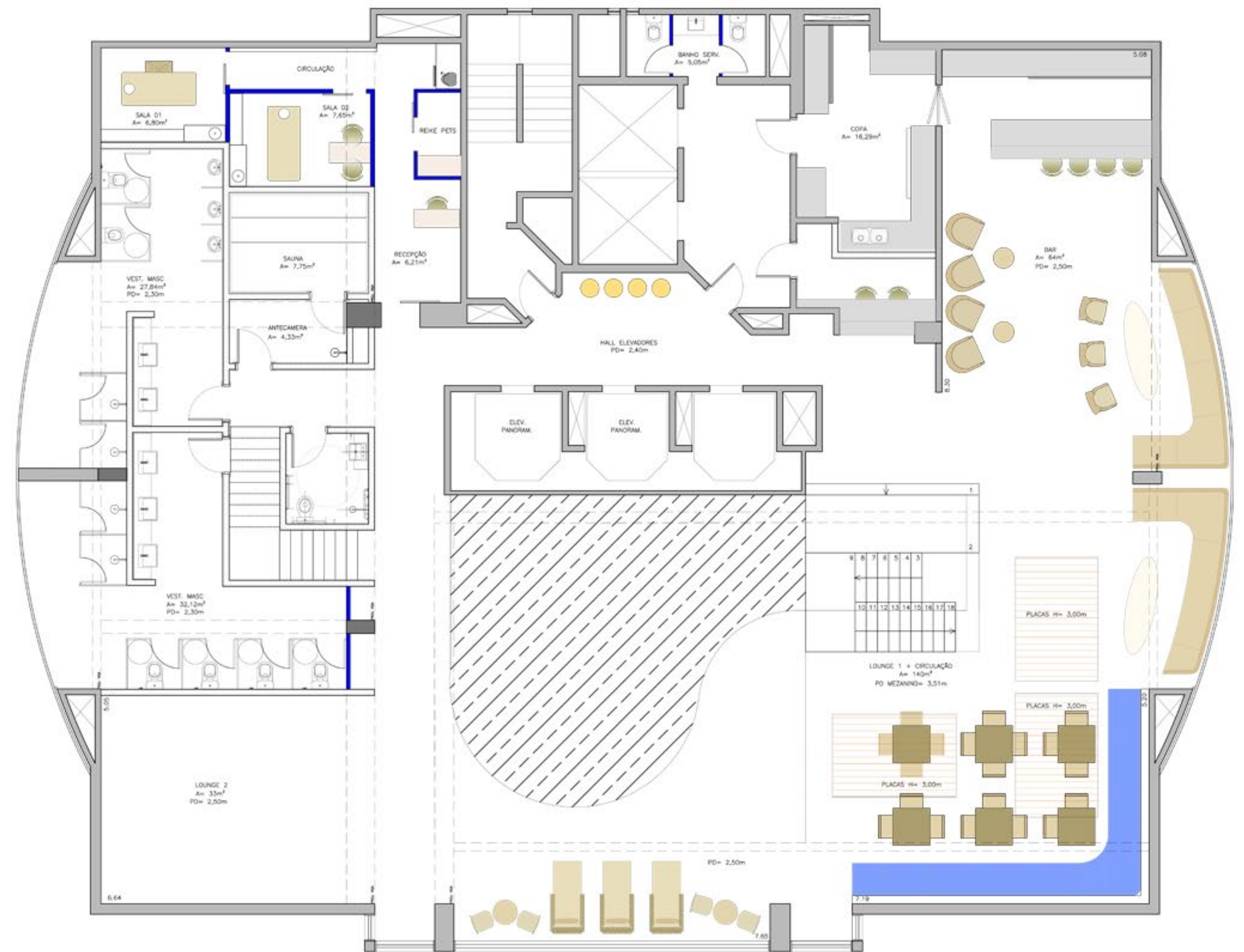
PLANTA NÍVEL PISCINA ESCALA 1:50
